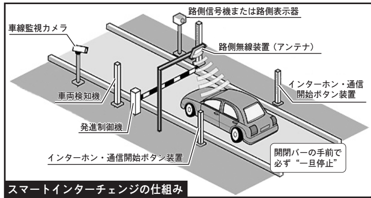
スマートインターチェンジの仕組み
